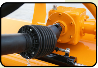
► Roue libre sur cardan
